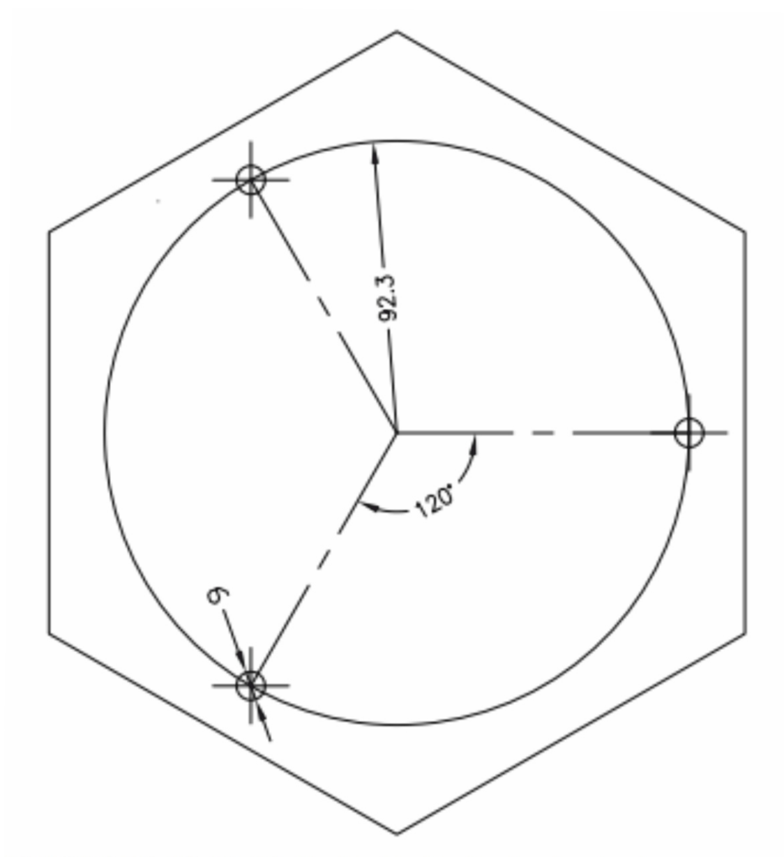
ESQUEMA DE LA BASE 060J-060D-060E
