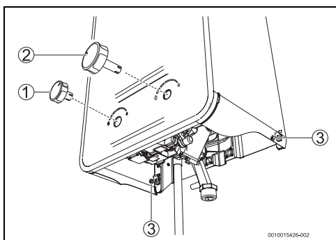
Fig. 13 Retirar la carcasa
