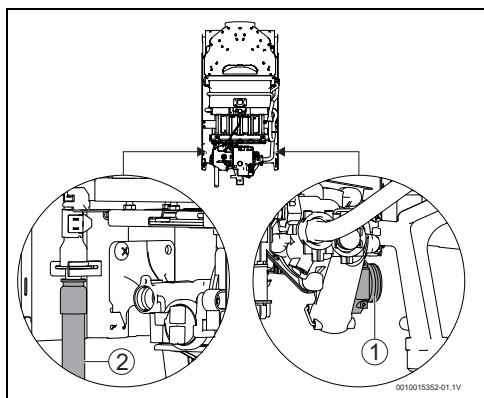
Fig. 10 Conexión de agua
