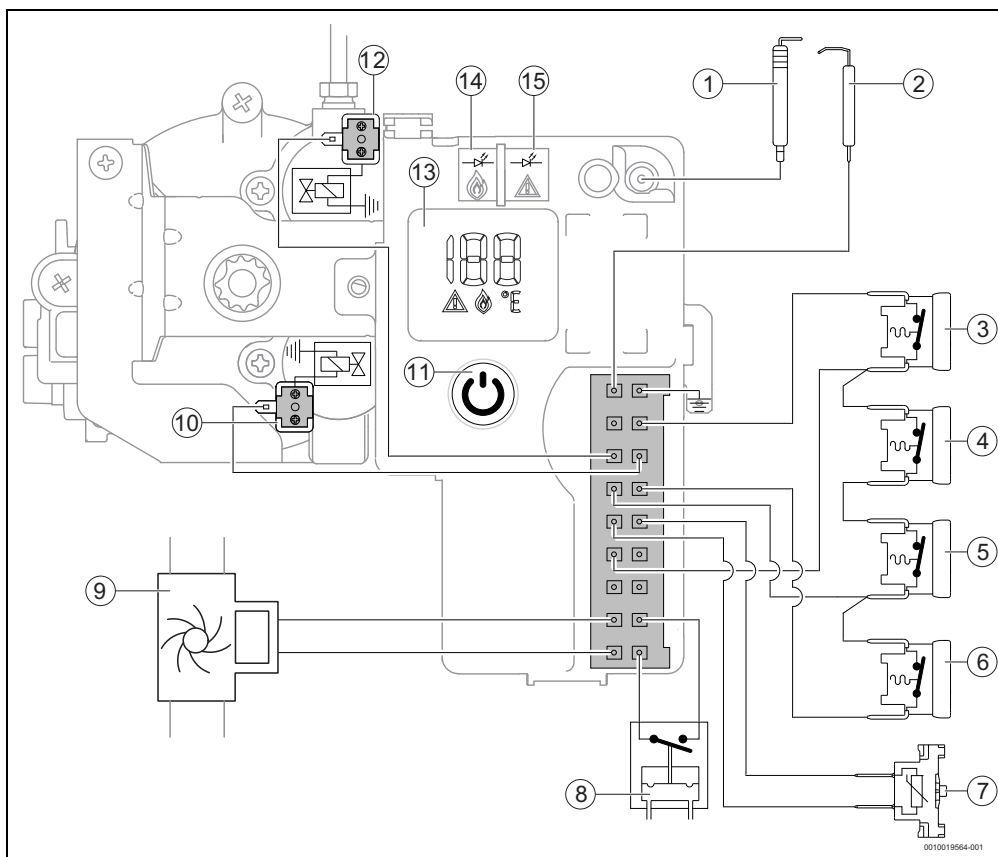
Fig. 27 Esquema de conexión
