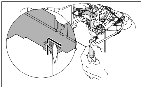
Fig. 25 Resetear el microinterruptor
