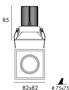
511D + HLX08
