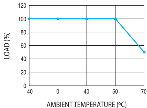
Potencia de salida - Temperatura
