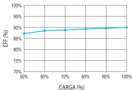
Eficiencia
