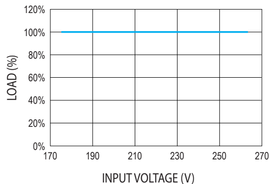
Potencia de salida - Tensión de entrada
