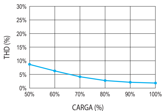
Distorsión Armónica
