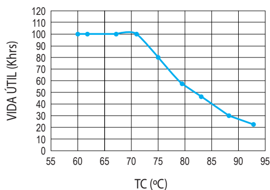
Vida Útil
