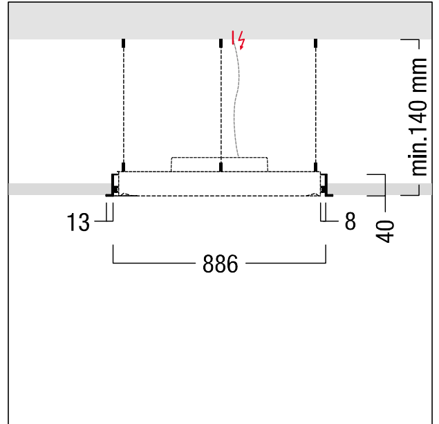
ZS_OND_M_870LED_Einbau.wmf
