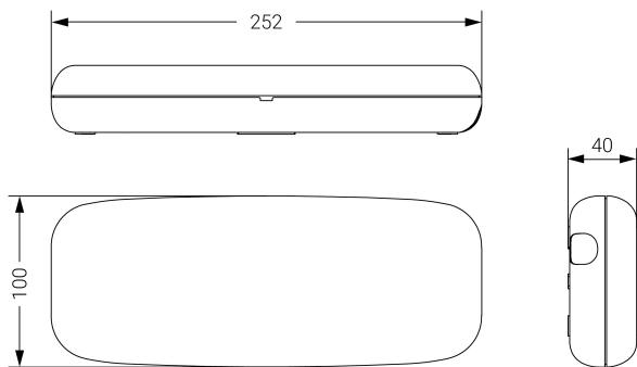
Dimensiones (mm):
