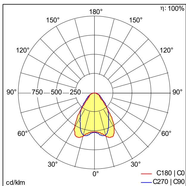
D35001_TECTON_C_3700-835_L1000_WB_LDE_WH.Idt
