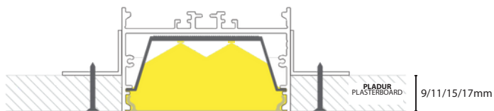
Fijación con aleta Mounting with flap
