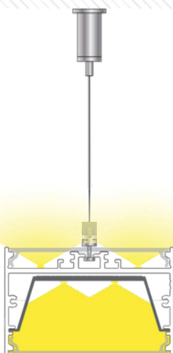
Fijación con tensor y doble difusor (Up&Down) Mounting with tensioner and doble diffusor (Up&Down)
