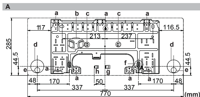
A Placa de montaje para la clase 20~35 a Puntos de fijación recomendados para la placa de montaje b Cavidad para la cubierta del orificio de la tubería c Pestañas para colocar e nivel d Orificio de paso Ø65 mm e Posición del tubo flexible de drenaje f Posición de la cinta métrica en el símbolo ">" g Extremo de la tubería de gas h Extremo de la tubería de líquido
