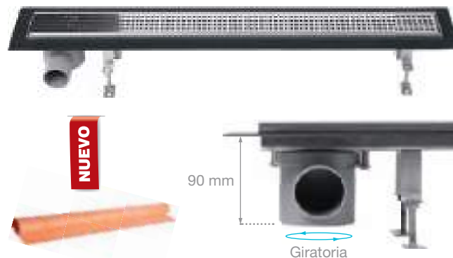
Canaleta Quadro 800 mm con válvula 75 mm · Fabricada en acero inoxidable AISI 304 · Válvula de 75 mm con salida a desagüe de Ø 50 mm
